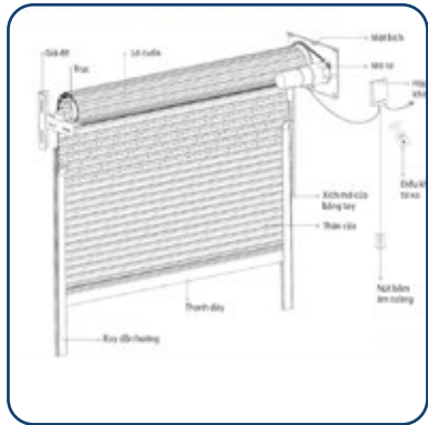
Mô Tơ Motor
